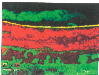
Abb. 2 Elementverteilungsbild vom Anschlag der Grundplatte.
